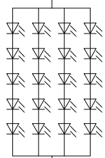
电路图 (5串4并)
