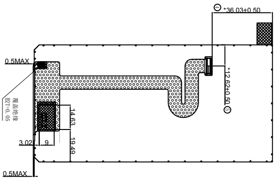
FPC折弯示意图 折弯出货
